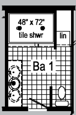
Optional 4'x6' Walk-In Tile Shower (omits linen)
