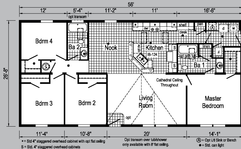
Optional Stairwell
